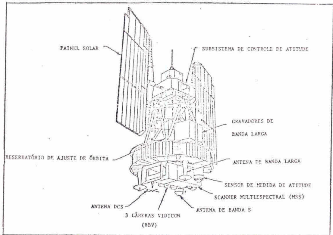
Fig. 2.2 - Configuração do satélite LANDSAT.
